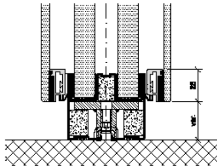
Bodenanschluss
