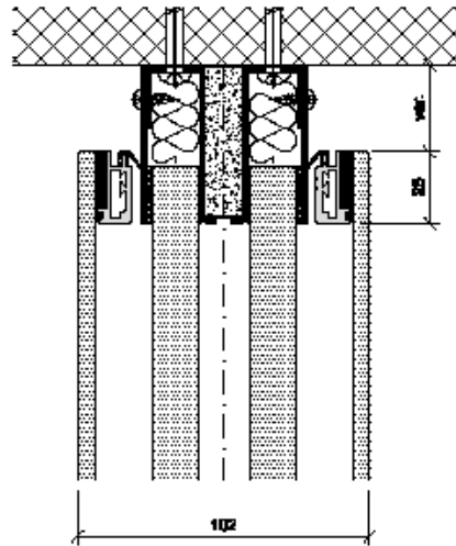
Deckenanschluss
