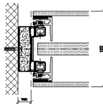
Anschluss variabel
