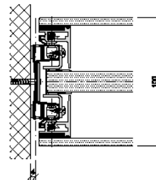
Wandanschluss
