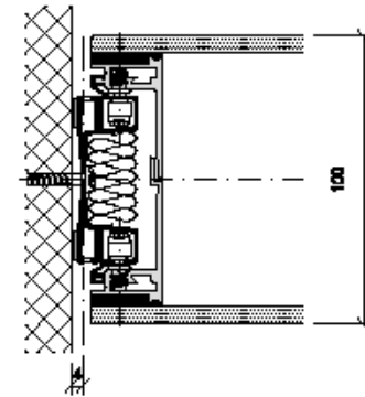
Wandanschluss
