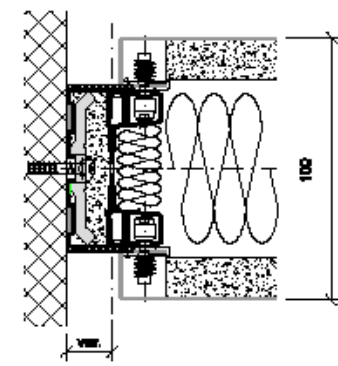
Anschluss variabel
