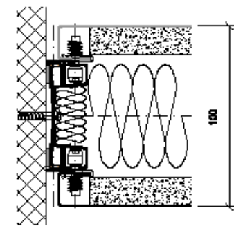
Wandanschluss
