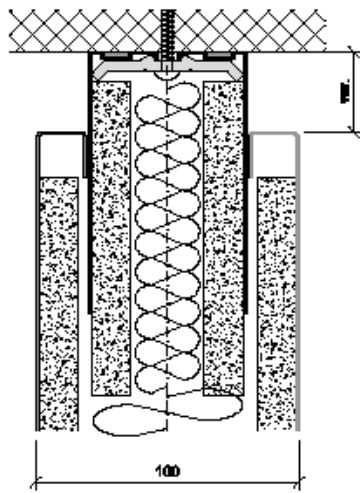
Deckenanschluss
