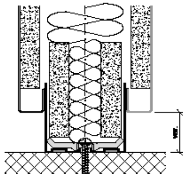
Bodenanschluss
