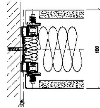
Anschluss Anfangsfuge
