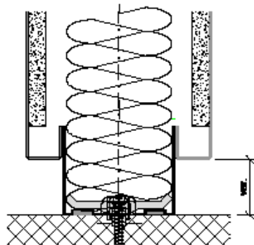
Bodenanschluss
