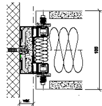
Anschluss variabel
