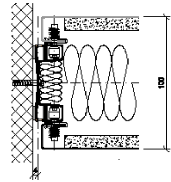
Wandanschluss
