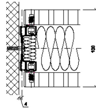
Anschluss variabel
