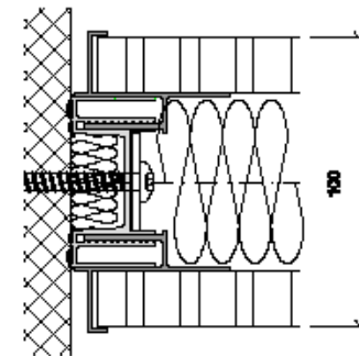
Anschluss Passprofil
