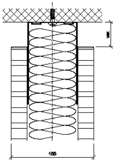
Deckenanschluss
