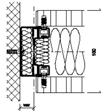
Anschluss Passprofil
