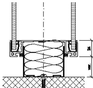
Bodenanschluss
