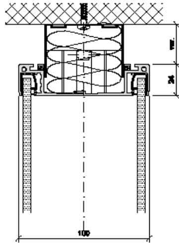
Deckenanschluss
