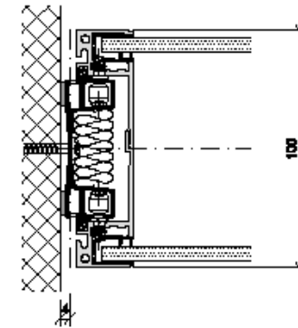
Anschluss Anfangsfuge
