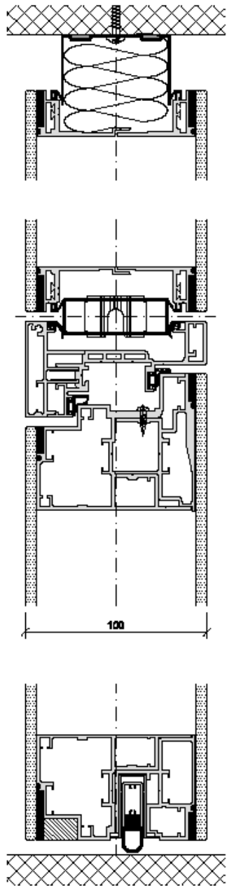
Vertikalschnitt
