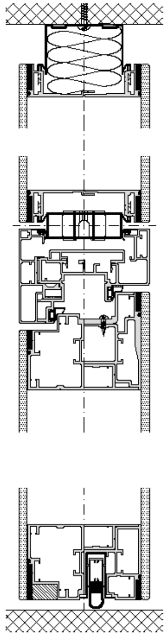
Vertikalschnitt
